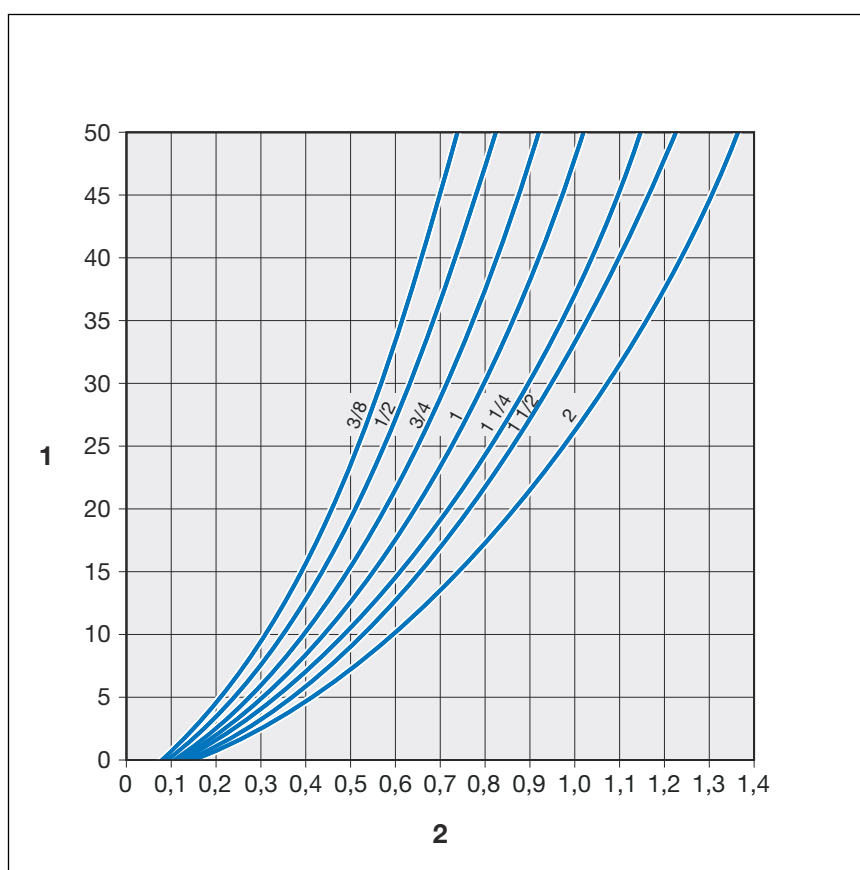
sl. 7: Upogibni krak v obliki črke U za Megapress \frac{3}{8} do 2 coli
