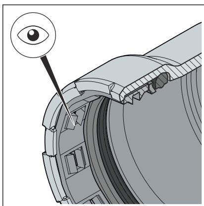
sl. 15: reznalni obroček
