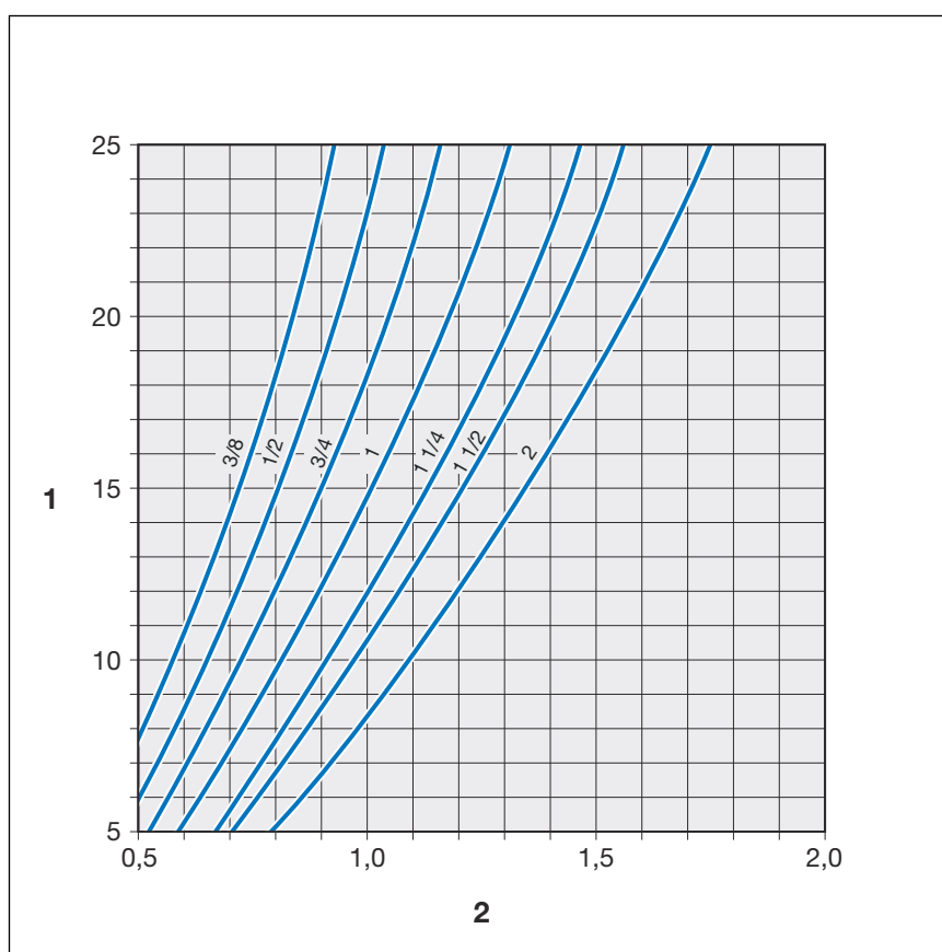
sl. 5: Upogibni krak v obliki črke Z in T za Megapress ¾ do 2 coli
